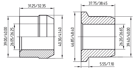
ERSC32G 25.4mm Standard
